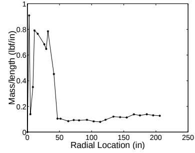
(d) Weight per unit length distribution.
